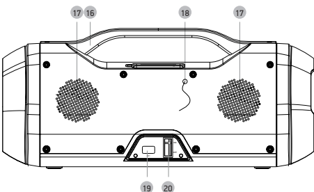
Задняя панель
