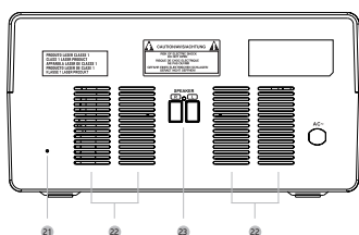
Задняя панель основного блока
